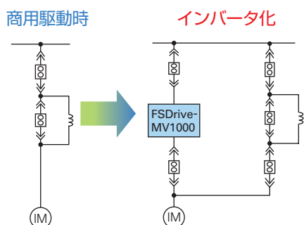
(例1) 商用バックアップシステム
