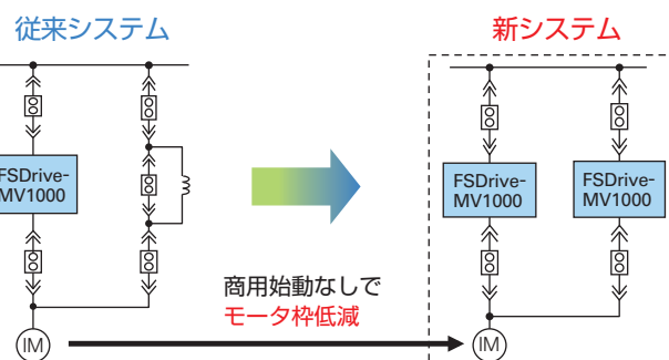
(例2) インバータバックアップシステム
