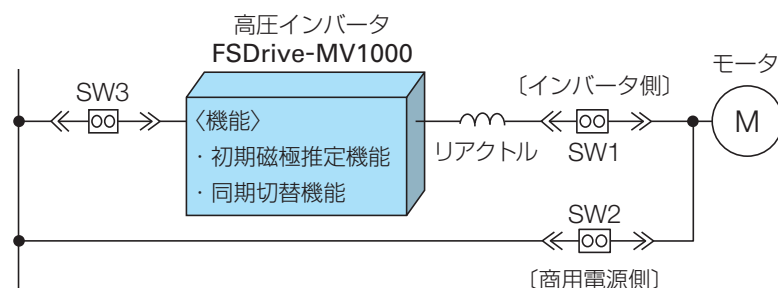
(例4) 同期モータの同期切替システム
