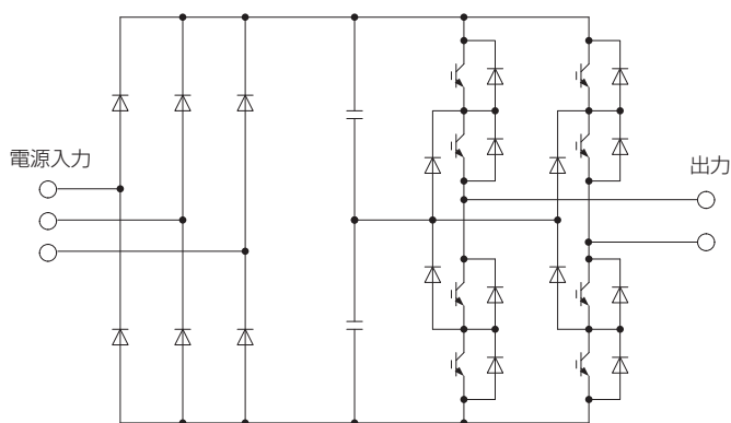
● パワーセル (1 個) の構成
