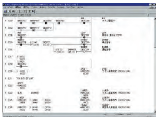
▲ラダープログラム
