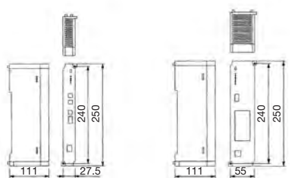
1スロット幅モジュール
