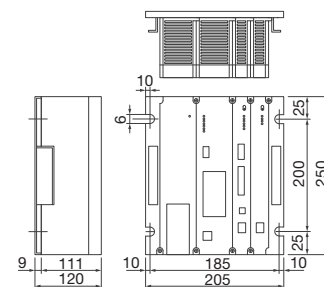
ショートマウントベース (MB-05)
