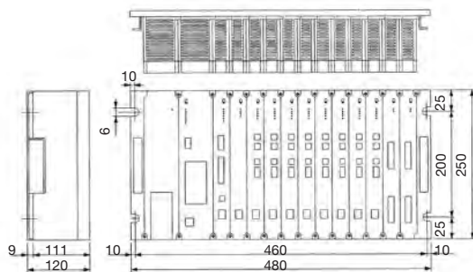
ロングマウントベース (MB-01)
